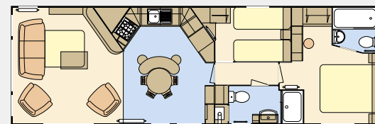
SFD layout
