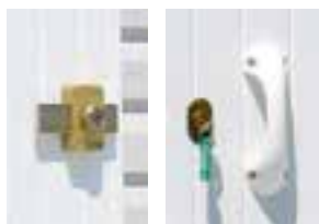
Porte PVC (1,73 x 0,81 m) avec ferrage aluminium blanc monté sur gonds polyamide. Verrou de sécurité en laiton + 3 clés.
