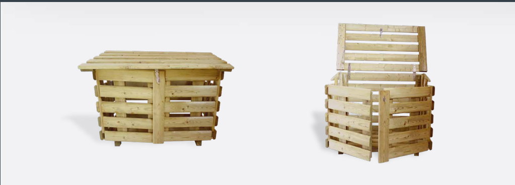
CACHE-GAZ Lg : 1,00 m, pour 2 bouteilles, dessus et façade ouvrantes, porte-cadenas, avec plancher et fond. Larg 0,53 m x H 0,85 m/0,74 m x Lg 1,04 m
